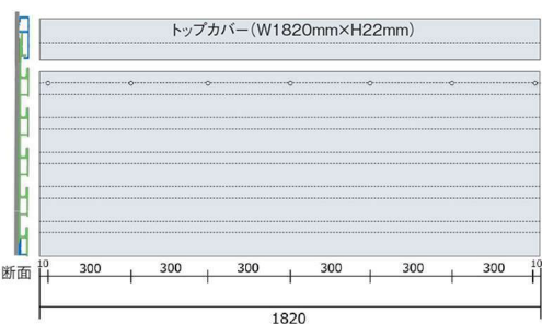
メディカルウォール (W1820mm×H150mm) 本体150mm+トップカバー取付高13mmとなります。
